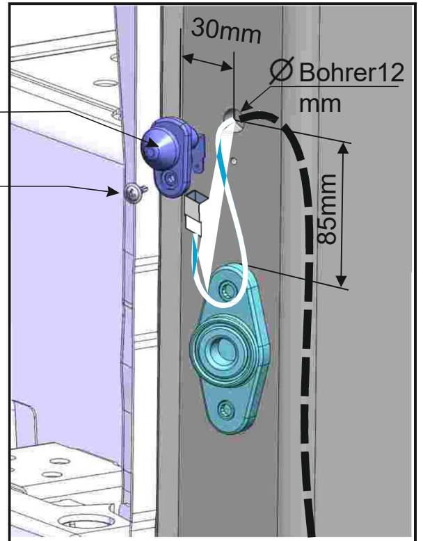
B-Säule
